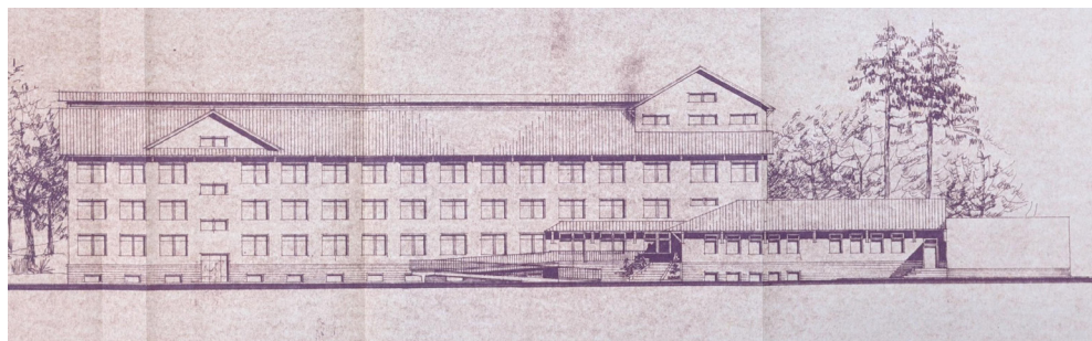
Ryc. 12. Projekt fasady południowej budynku B. II. Chrzanowicz, B. Grodź, 1984. DPS, sygn. DT/292
